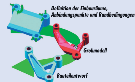
Topologieoptimierung eines Bauteils
