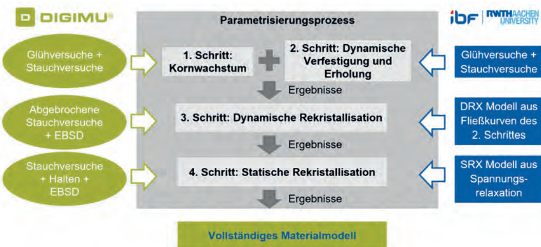
Bild 2: Charakterisierungs- und Parametrisierungsprozess in DIGIMU® (links) und angepasst durch das IBF (rechts)
